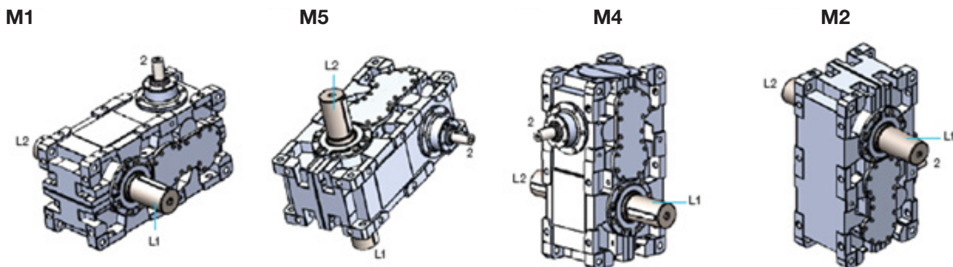
Figura 5 - Posições de montagem
