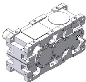
Pés / carcaça
