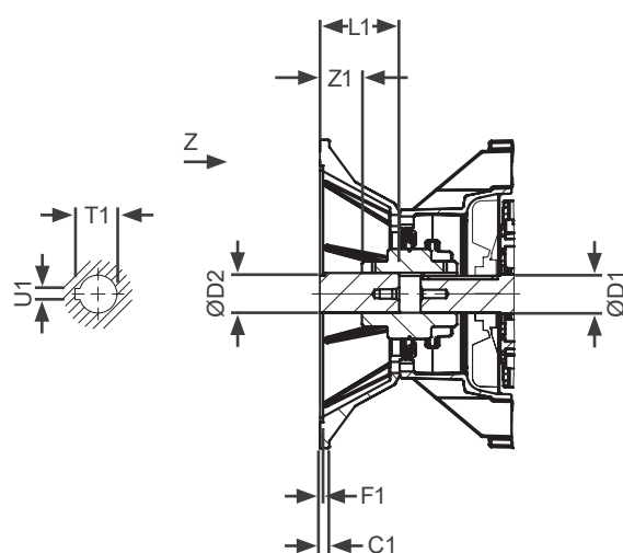
Detalle Y
